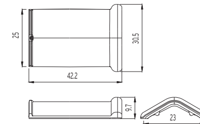
4 WALMKAPPE 4-SEITIG
