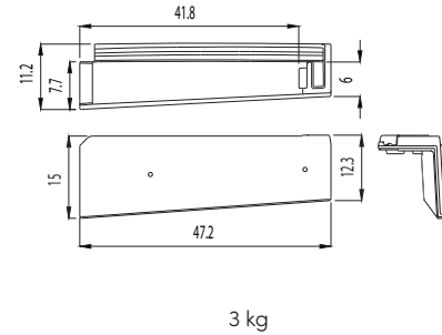
14 DURCHGANGSZIEGEL FLAT-5XL
