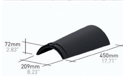
4 WALMKAPPE 3-SEITIG RUND
