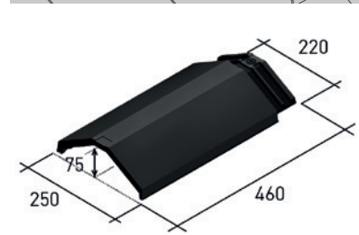
5 WALMKAPPE RUND 4-SEITIG
