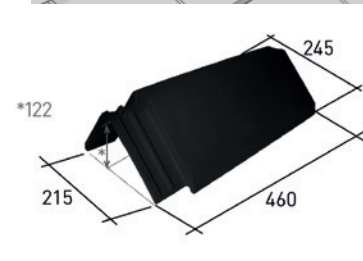
6 WALMKAPPE ECKIG 3-SEITIG
