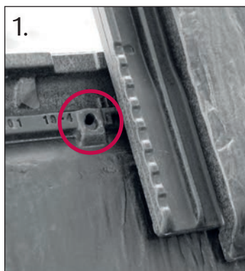
Dachziegel auflegen.
