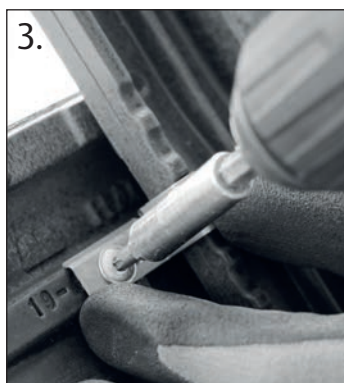
Klammer anschrauben.
