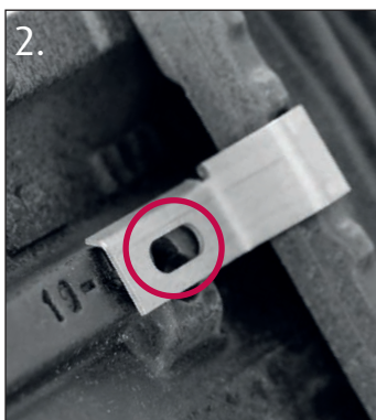
Kopf-Seitenfalzklammer positionieren.
