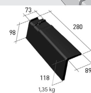
17 DUNSTROHRZIEGEL
