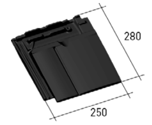
18 LÜFTERZIEGEL
