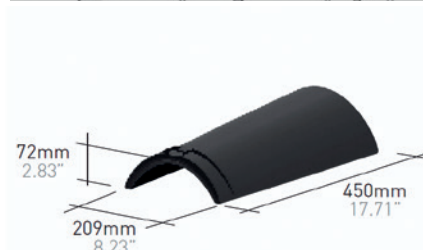
4 WALMKAPPE 3-SEITIG RUND
