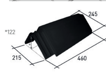
6 WALMKAPPE ECKIG 3-SEITIG
