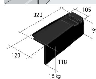
16 HALBER ZIEGEL RECHTS
